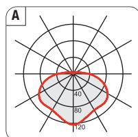
curva fotometrica_photometric data
