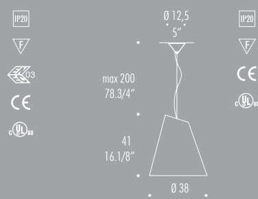
MICENE S38 AL max 1x150W- 250V E27
