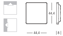
6949 anodizzata/anodized
