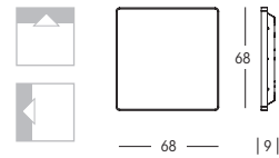
6950 anodizzata/anodized
