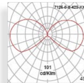
TC-D G24d-2 18W
