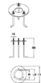
599.9030.A.00.00.Z Base di ancoraggio Anchor bolt kit
