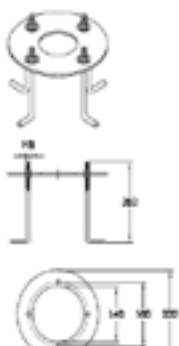
599.9031.A.00.00.Z Base di ancoraggio Anchor bolt kit
