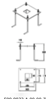
599.9032.A.00.00.Z Base di ancoraggio Anchor bolt kit
