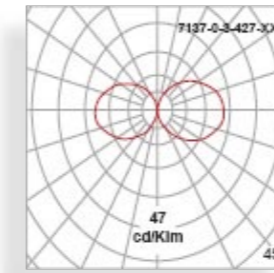
TC-D G24d-2 2x18W
