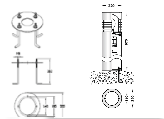
599.9031.A.00.00.Z Base di ancoraggio Anchor bolt kit
