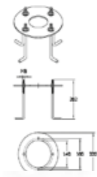
599.9031.A.00.00.Z Base di ancoraggio Anchor bolt kit
