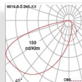
QT32 E27 60W
