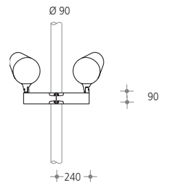
OLIVIO Medio SX 811 Double lateral projector
