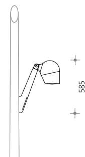
OLIVIO Medio SX 779 Straight arm
